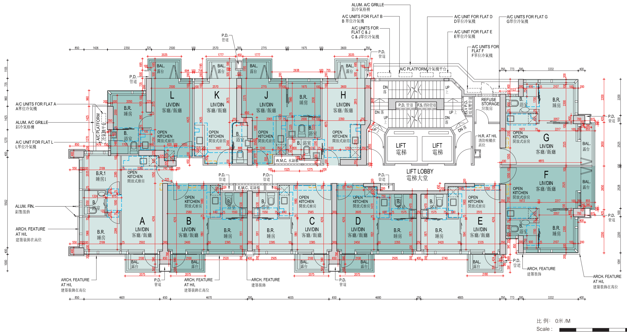
31樓平面圖 31/F Floor Plan
